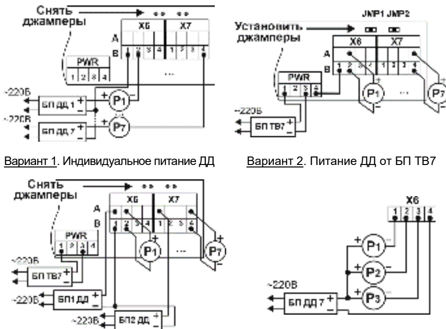
Вариант 4. Подключение ДД к ТВ7-04.1М Лайт
