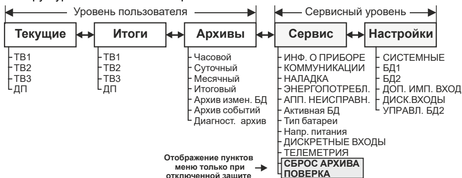
Рис. 2.6 – Структура меню тепловычислителя
