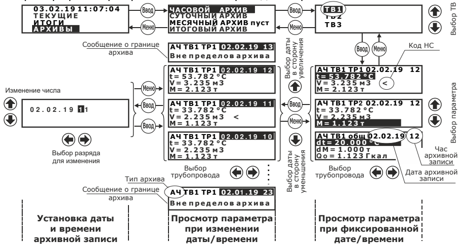
Рис. 3.7 – Примеры вывода на индикатор архивных величин
